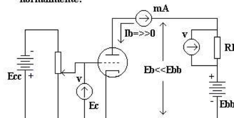
(C) Grade próxima de zero: I_b \Rightarrow \gg 0 e queda de tensão sobre RL grande. A tensão de placa E_b é bastante inferior a E_{bb} . Triodo perto da saturação.
