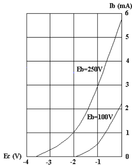
Curvas características de transferência duplo-tríodo ECC83
